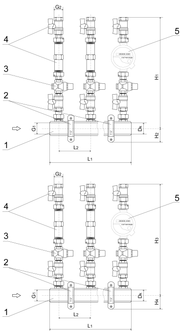
Устройство коллекторного модуля
